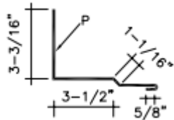
Side Wall SW1
