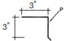
Eave Drip EF3
